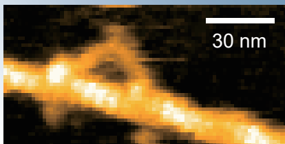
Walking Myosin V N. Kodera et al. Nature 2010.
