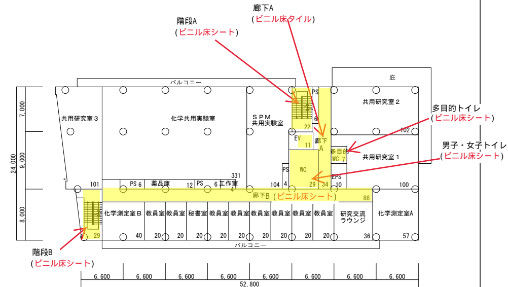
3階平面図 S=1/600 1,319㎡
