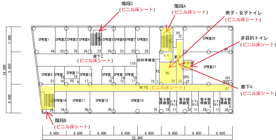
地下1階平面図 S=1/600 1,286㎡
