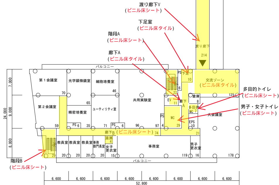
4階平面図 S=1/600 1,319㎡
